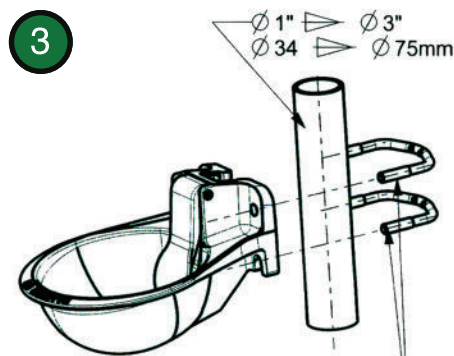
KIT A-315 : Ø 1" ➤ Ø 2" KIT A-316 : Ø 2" ➤ Ø 3"
